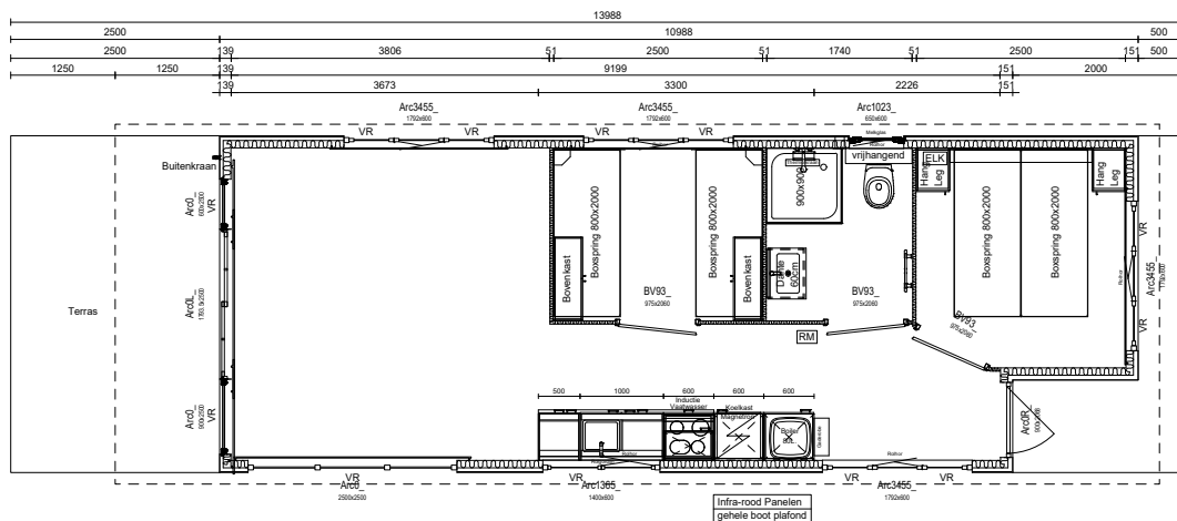
Plattegrond
